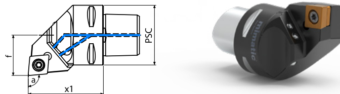
Spannschraube Screw clamp
