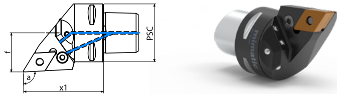
Kniehebelspannung Lever-look clamp
